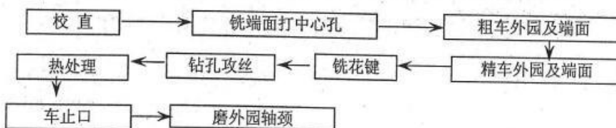
图2 机加车间工艺流程
