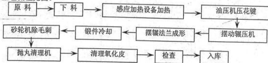
图1 锻造车间工艺流程
