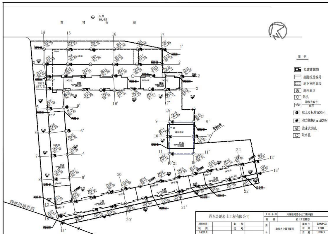
图 3-2 河畔明珠 C 区勘察 钻孔平面图
