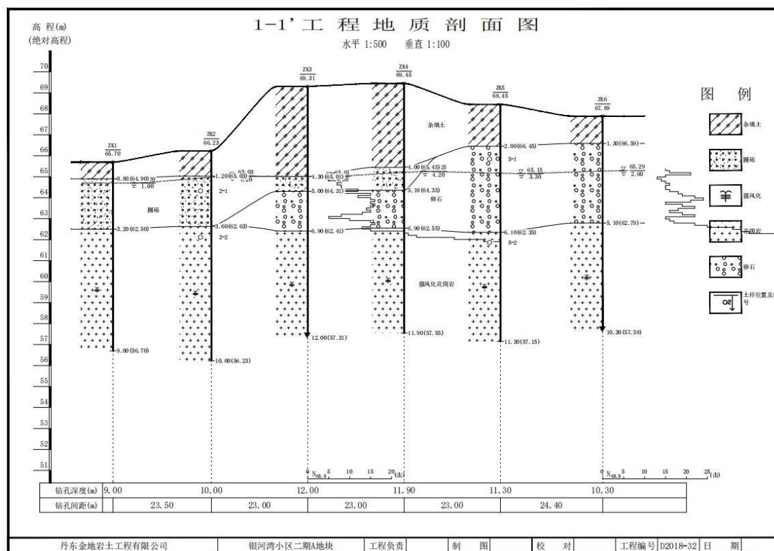
图 3-3 工程地质剖面图
