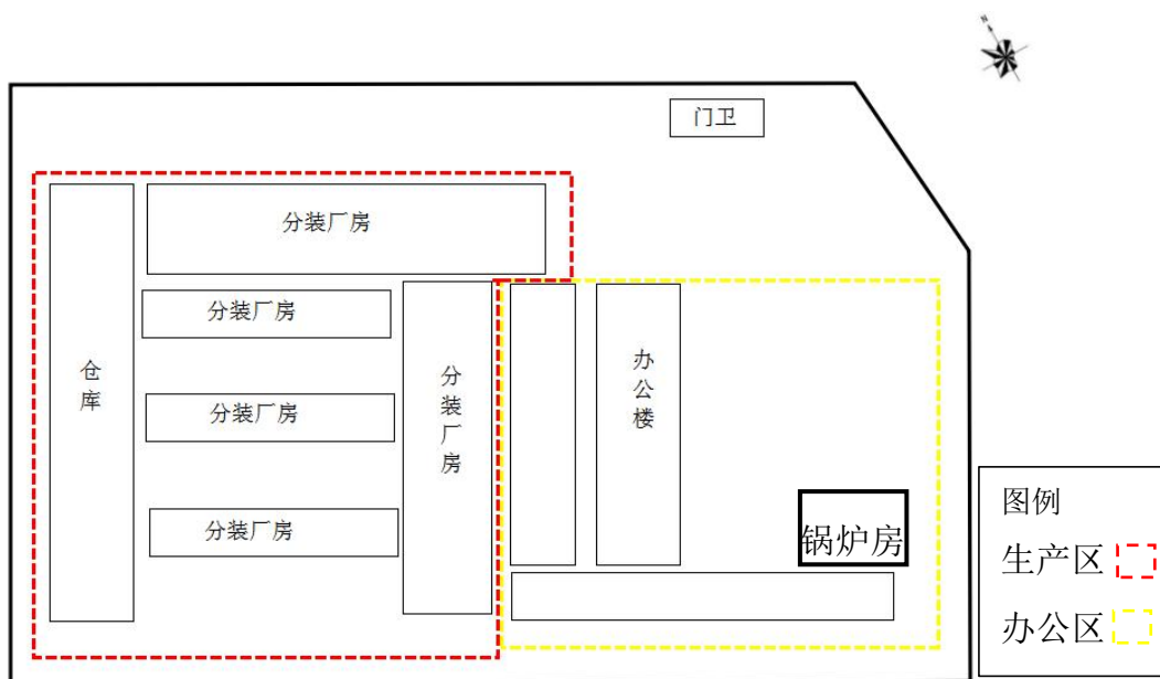
图 3-15 厂区平面布置图
