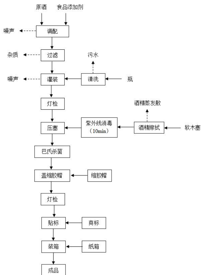
图 3-16 工艺流程图
